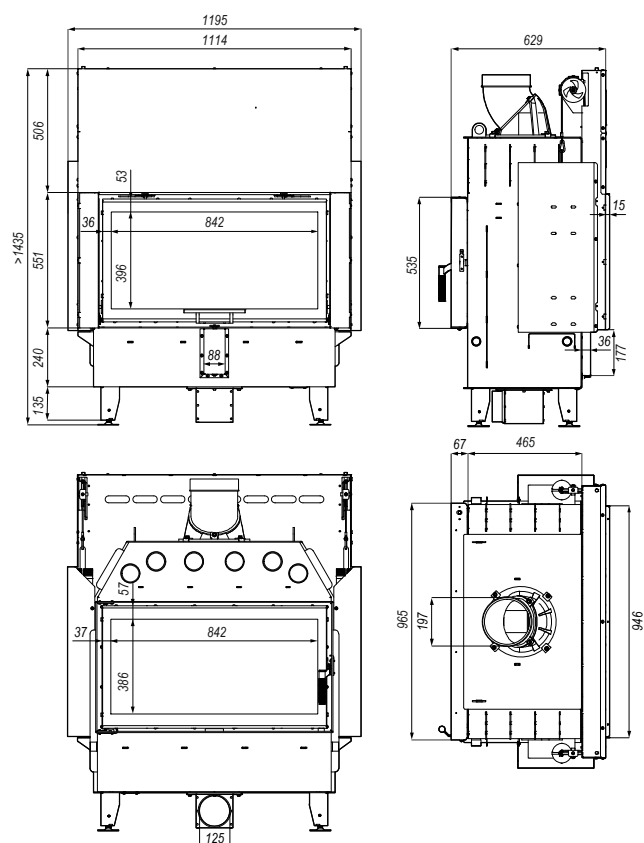
Rysunek 35. Wymiary wkładu kominkowego DEFRO HOME INTRA LA T G.
