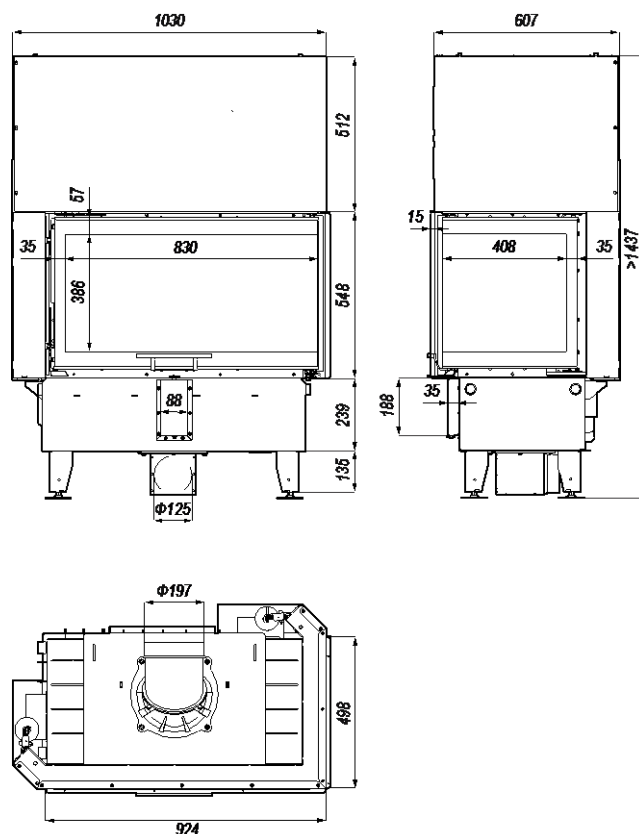
Rysunek 27. Wymiary wkładu kominkowego DEFRO HOME INTRA ME BP G.
