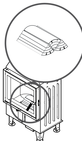
Rysunek 42. Sposób ułożenia paliwa
