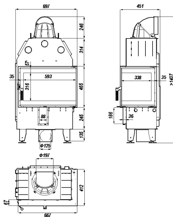
Rysunek 22. Wymiary wkładu kominkowego DEFRO HOME INTRA SM BP MINI.
