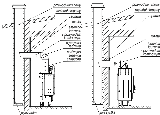
Rysunek 40. Podłączenie wkładu kominkowego do przewodu kominowego w zależności od wersji (z lewej wersji XSM i XLA, z prawej pozostałe).
