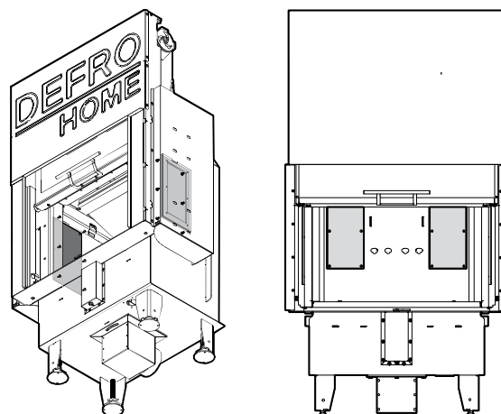
Rysunek 50. Umieszczenie pokryw otworów rewizyjnych we wkładach: DEFRO HOME INTRA wersji G (po lewej) i DEFRO HOME INTRA wersji C G (po prawej).
