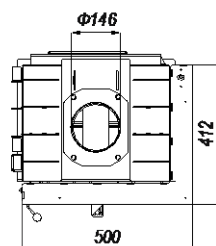
Rysunek 10. Wymiary wkładu kominkowego DEFRO HOME INTRA XSM BP MINI
