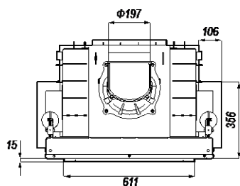
Rysunek 13. Wymiary wkładu kominkowego DEFRO HOME INTRA SM G
