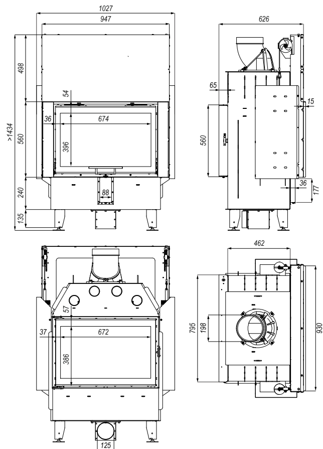
Rysunek 30. Wymiary wkładu kominkowego DEFRO HOME INTRA ME T G.
